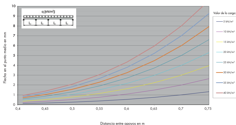
Flecha del tablero tricapa de 21mm
