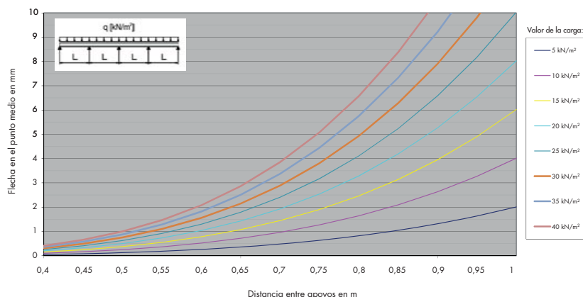
Flecha del tablero tricapa de 21mm
