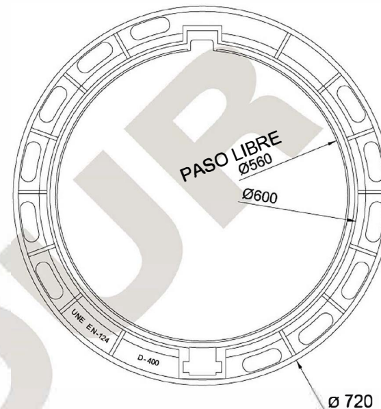
TAPA. SECCIÓN.
