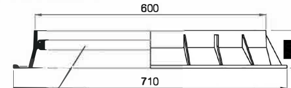
MARCO. SECCIÓN.
