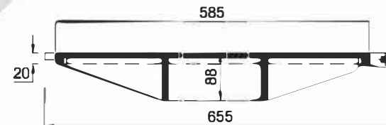
MARCO. SECCIÓN.
